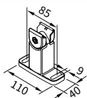
Supporto guida, regolabile in alto 100 mm
