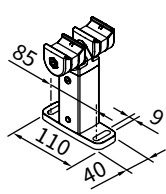
Supporto guide doppie, regolabili in alto 140 mm supporto centrale con 2 impianti singoli affiancati
