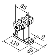
Supporto guide doppie, regolabili in alto 100 mm supporto centrale con 2 impianti singoli affiancati
