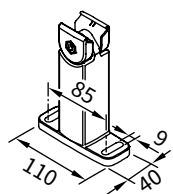
Supporto guida, regolabile in alto 140 mm
