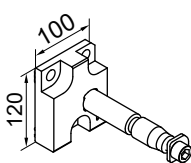
Supporto a parete lato destro
