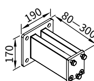
Distanziatore 80-300 mm
