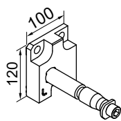
Supporto a parete lato sinistro
