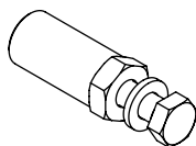
Riduttore M 16 → M 12 / SW 27
